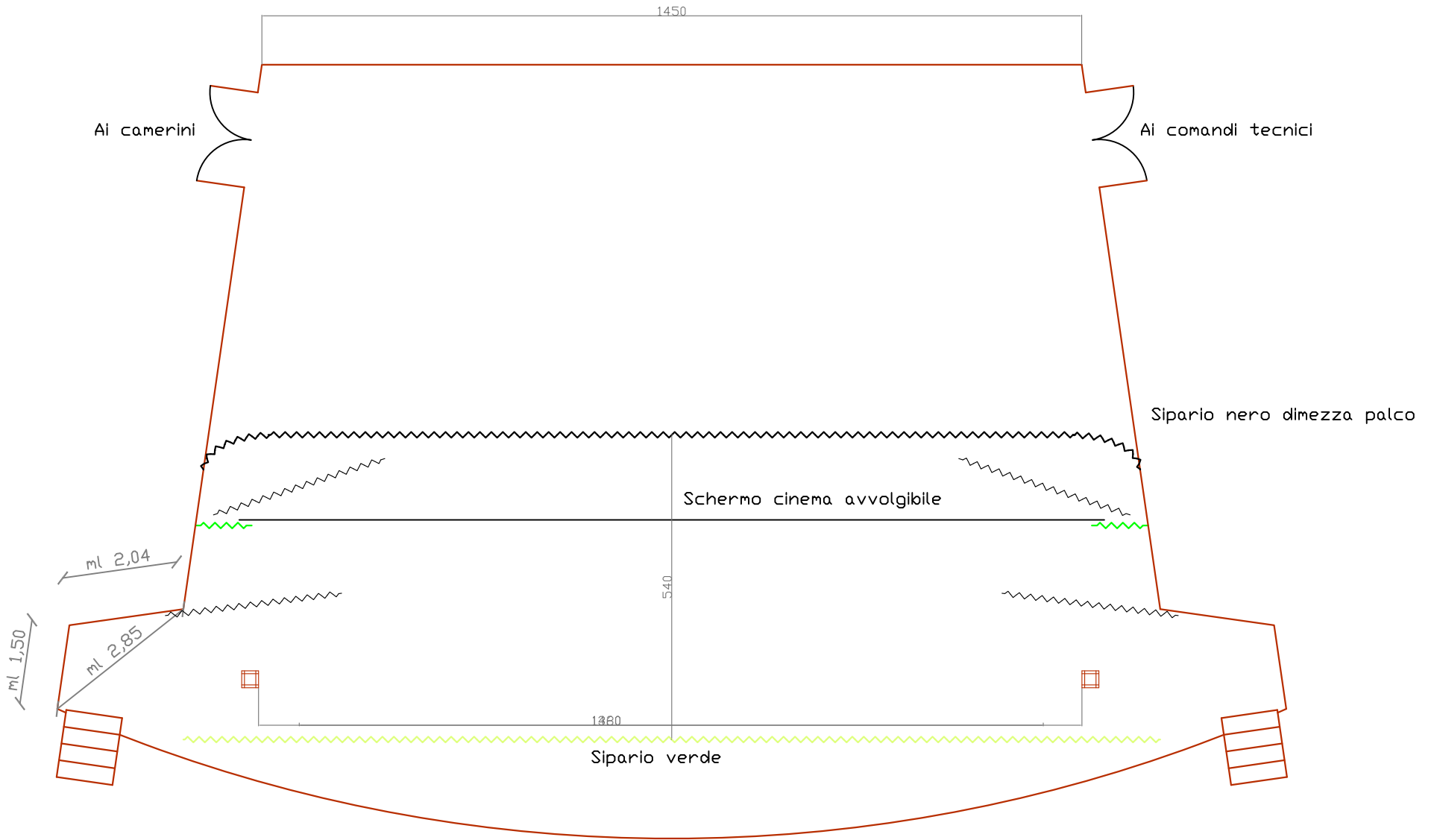
Configurazione a mezzo palco Quote spazi a terra
