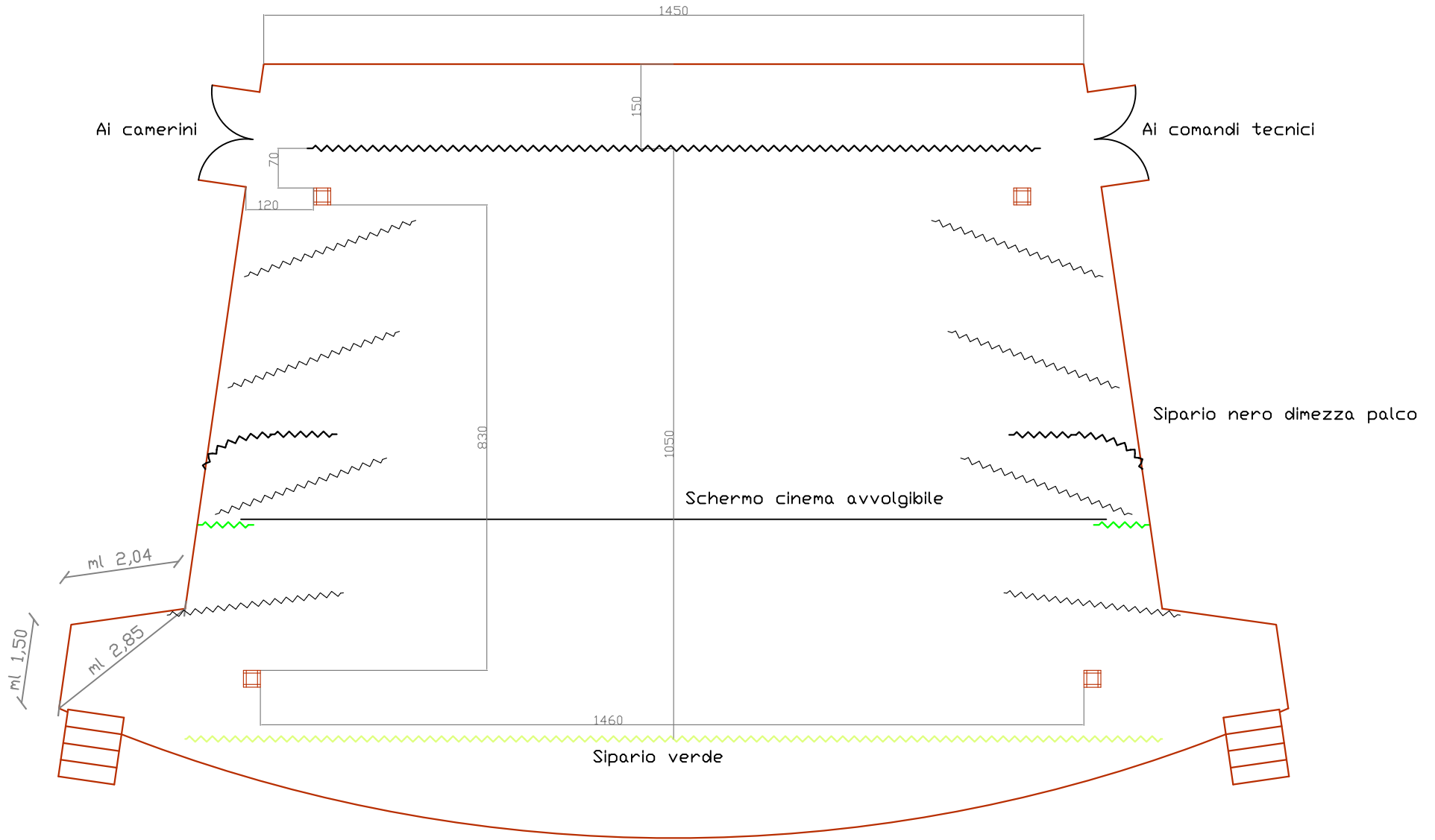
Configurazione a palco intero Quote spazi a terra
