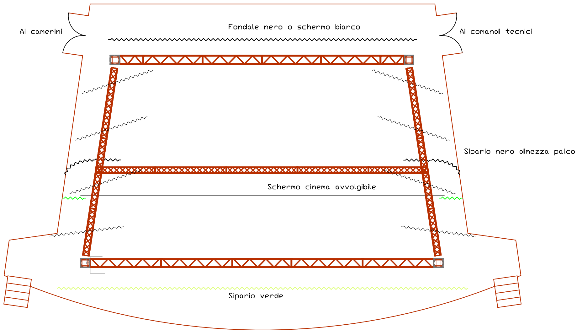
Configurazione a palco intero
