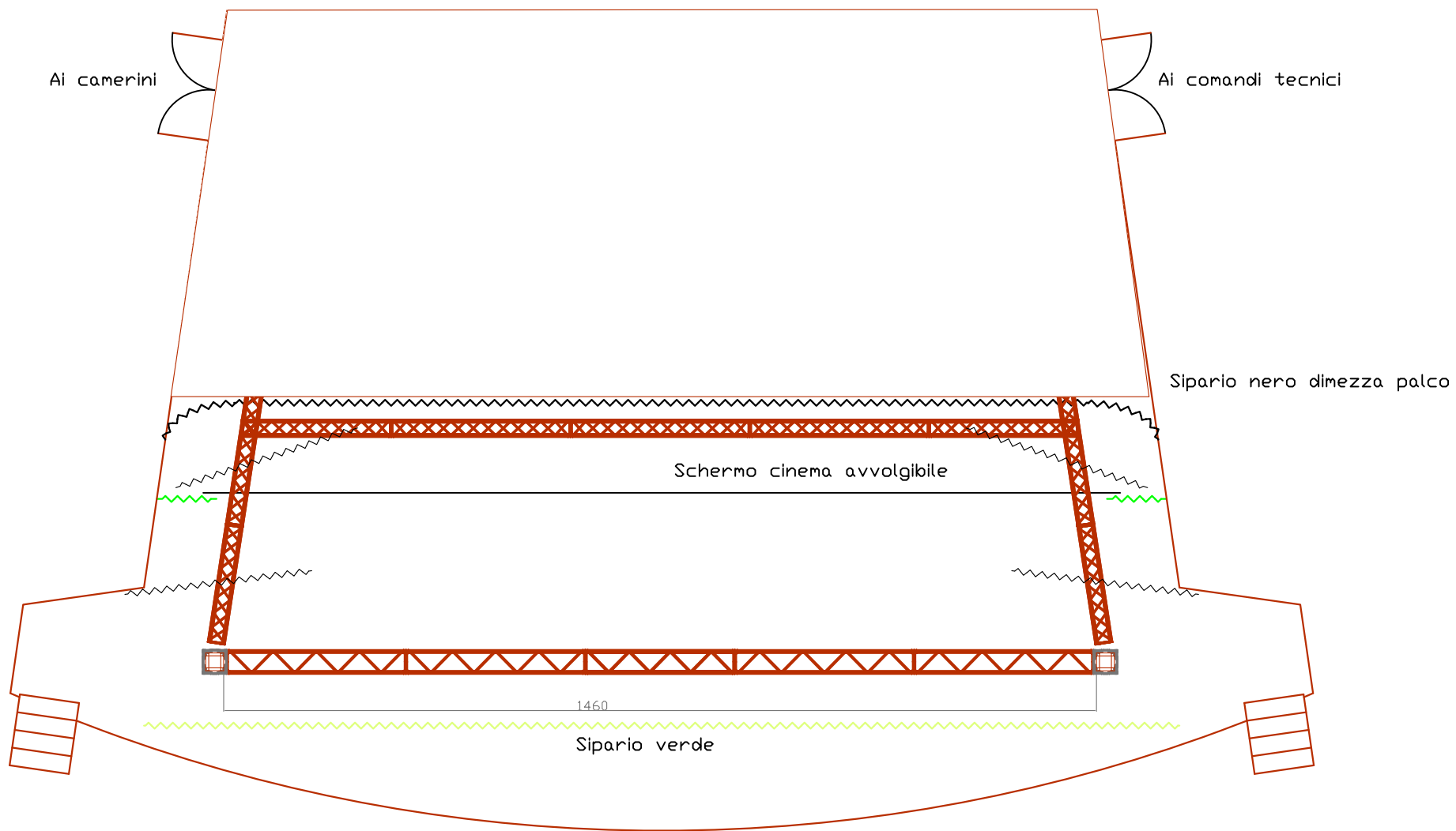
Configurazione a mezzo palco
